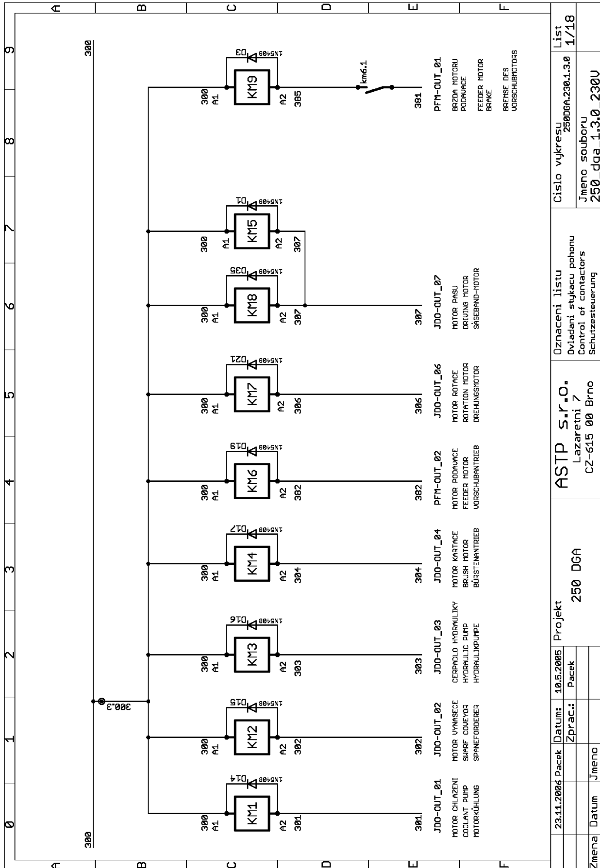
25.1. Elektrické schéma / Elektroschema / Wiring diagram 1
