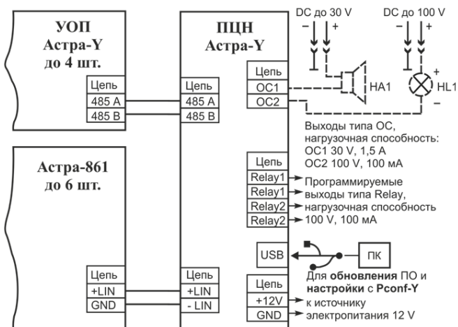
Схема подключения УОП к пульту «ПЦН Астра-У»
