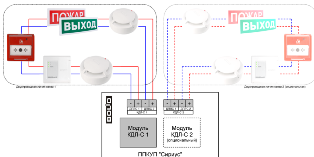
Рисунок 57. Схема подключения адресных устройств
