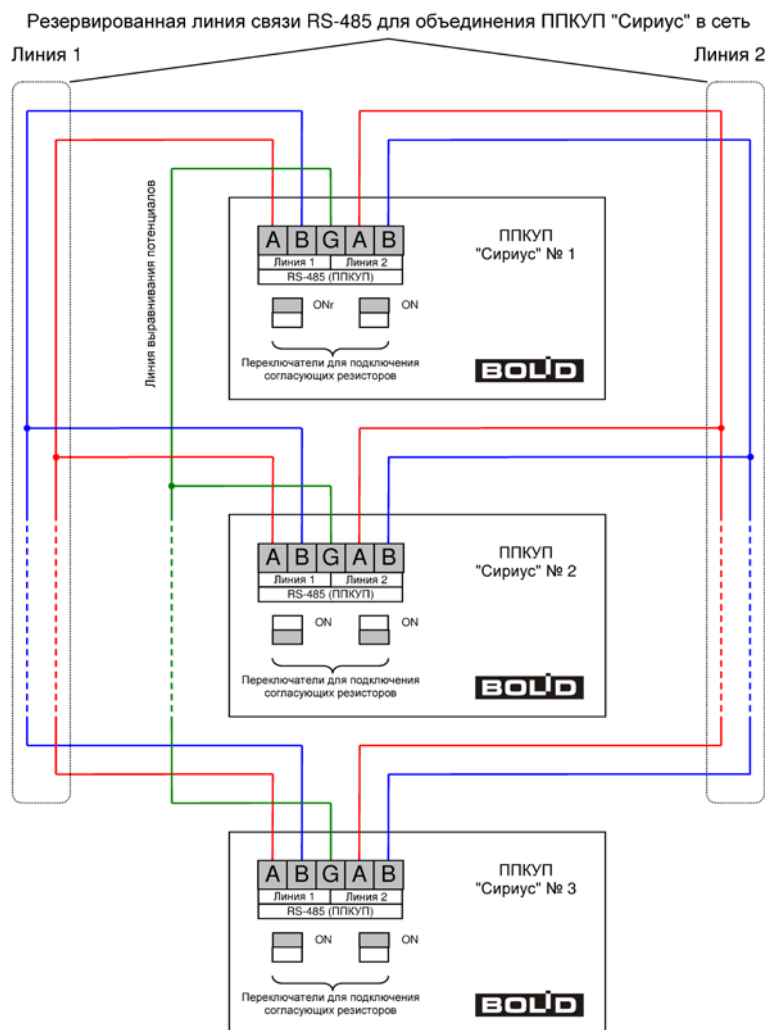
Рисунок 62. Схема объединения приборов «Сириус» в сеть
