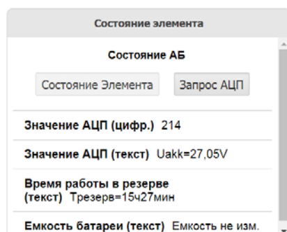
Рисунок 51. Отображение измеряемых величин на вкладке
