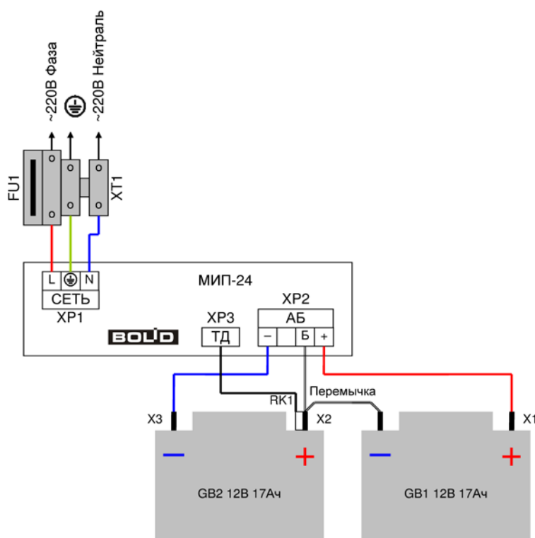
Рисунок 63. Схема подключения источников питания
