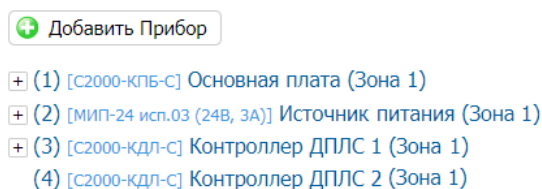
Рисунок 30. Список встроенных ведомых приборов
