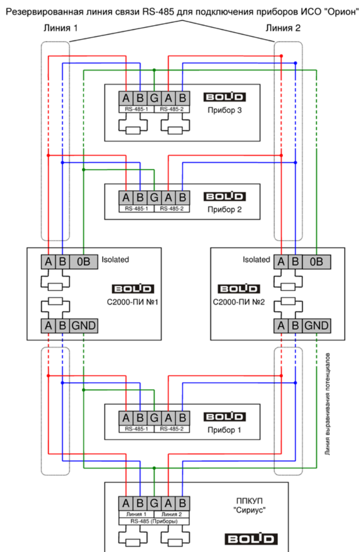
Рисунок 60. Схема подключения повторителей резервированного интерфейса RS-485 «C2000-ПИ»
