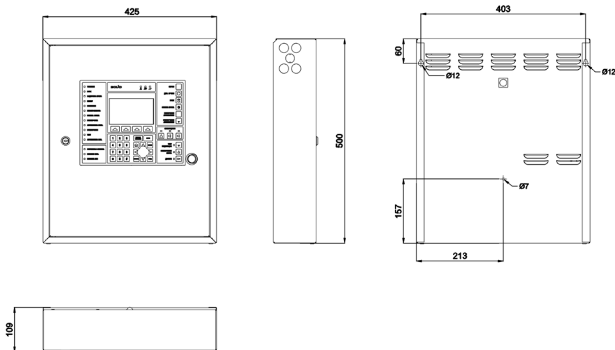
Рисунок 56. Габаритные и установочные размеры
