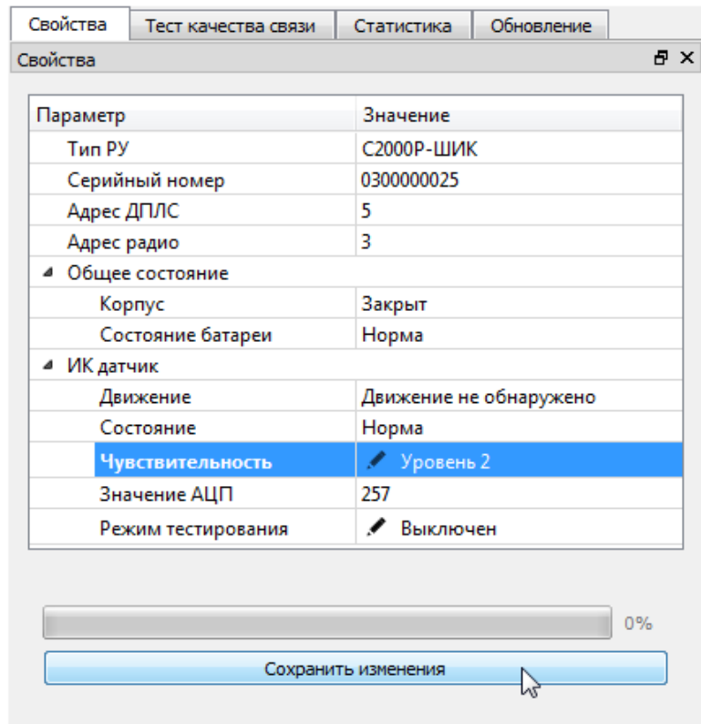
Рисунок 2.13 Настройка работы РУ
