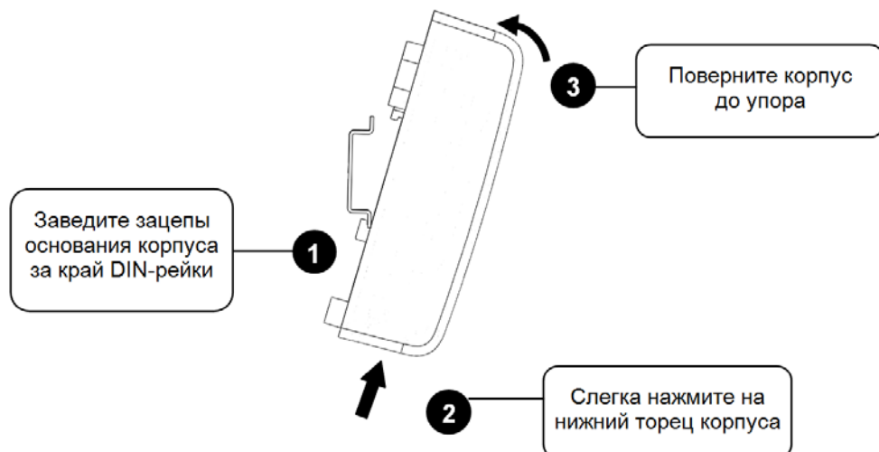
Рисунок 2.4 Монтаж на DIN-рейку
