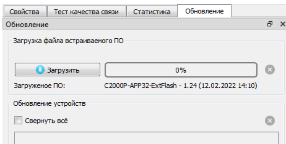
Рисунок 2.17 Вкладка «Обновление»
