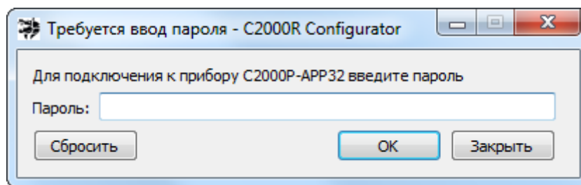
Рисунок 2.22 Запрос пароля
