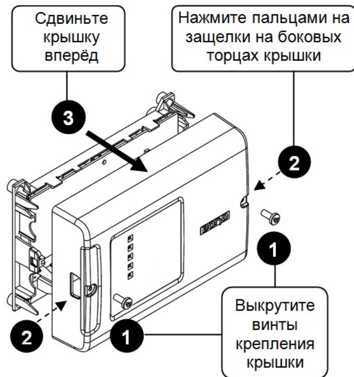
Рисунок 8-2 Снятие крышки
