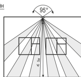
Г) Вариант установки на потолке
