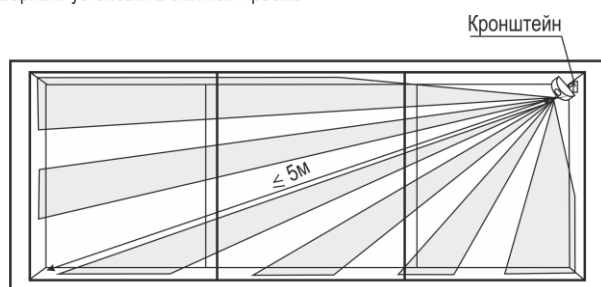
Д) Вариант установки между рамами
