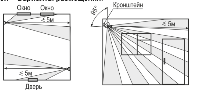
А) Вариант установки на стене (вид сверху)
