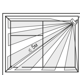
В) Вариант установки в оконном проеме
